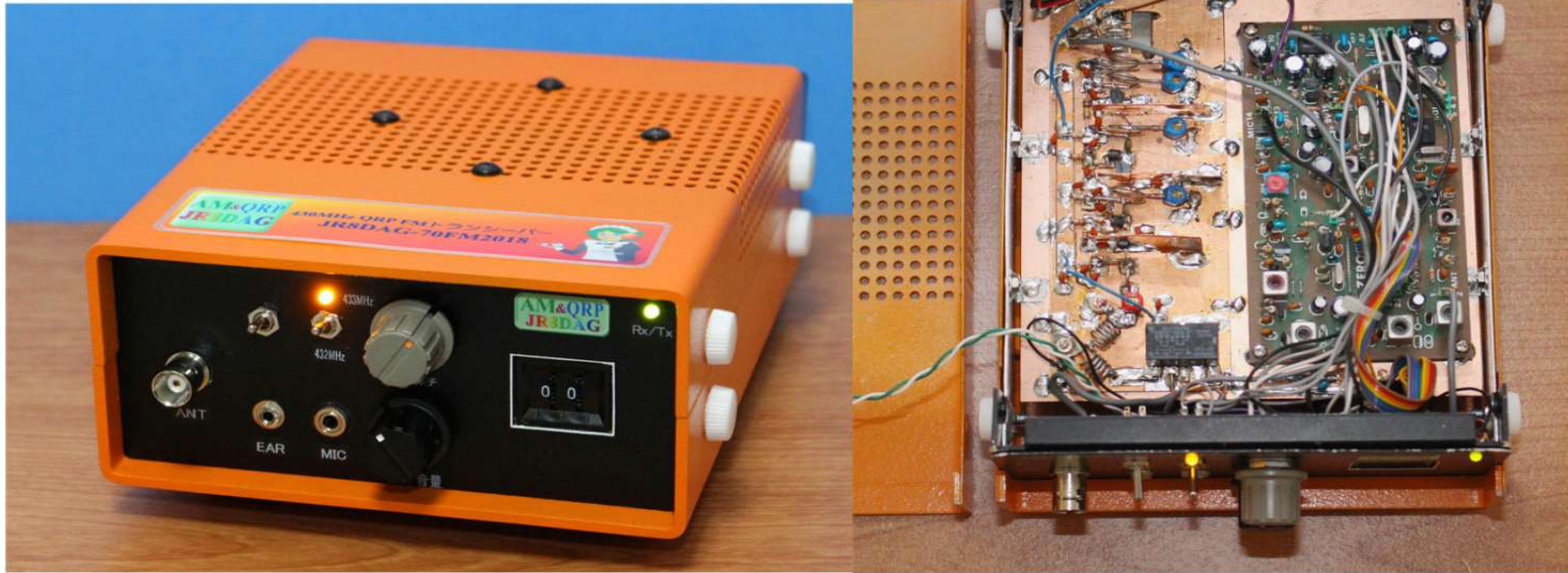
430Hz QRP FM トランシーバー (JR8DAG-70FM2018)
